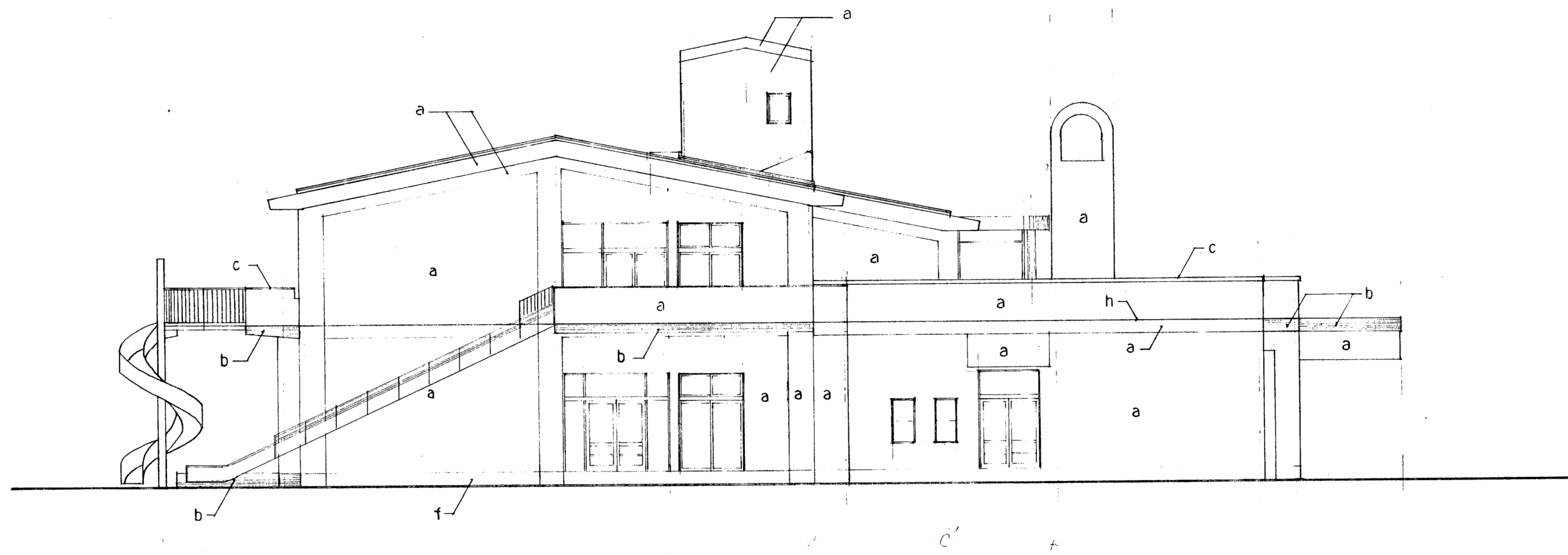
立面图 (东)
